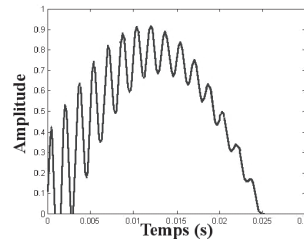
Figure 4. Force en fonction du temps.
