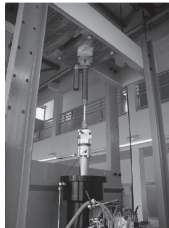
Figure 5. Vérin grande vitesse.
