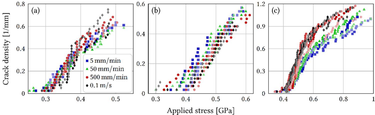
FIGURE 1 : ÉVOLUTION DU TAUX DE FISSURATION MATRICIELLE EN FONCTION DU CHARGEMENT APPLIQUÉ AU STRATIFIÉ POUR DIFFÉRENTES VITESSES DE CHARGEMENT ET DIFFÉRENTES CONFIGURATIONS DE STRATIFIÉS À PLIS CROISÉS : (A) [0/90 3 ]s, (B) [0/90 2 ]s ET (C) [0/90]s.
