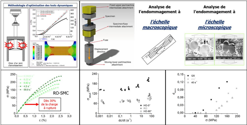
FIGURE 3 : CARACTÉRISATION MULTI-ÉCHELLE DU COMPORTEMENT MÉCANIQUE ET DE L'ENDOMMAGEMENT DES COMPOSITES ADVANCED-SMC SOUS SOLlicitATIONS DYNAMIQUES RAPIDES.
