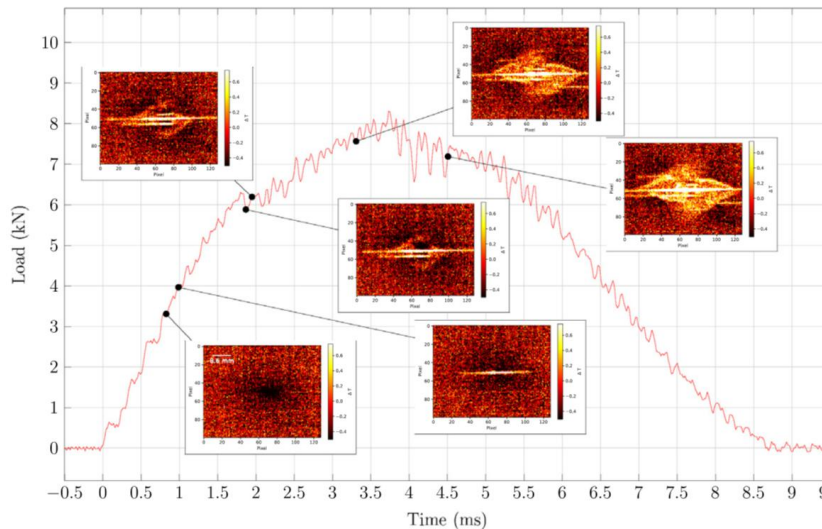
FIGURE 2 : ENDOMMAGEMENTS CAPTURÉS PAR THERMOGRAPHIE INFRAROUGE AU COURS D'UN ESSAI D'IMPACT BASSE VITESSE À 20J ET LIEN AVEC LE CHARGEMENT APPLIQUÉ À LA PLAQUE.
